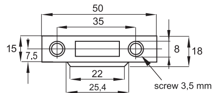
STRIKER PLATE
